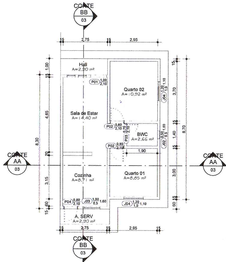
1 PLANTA BAIXA 1 : 100
