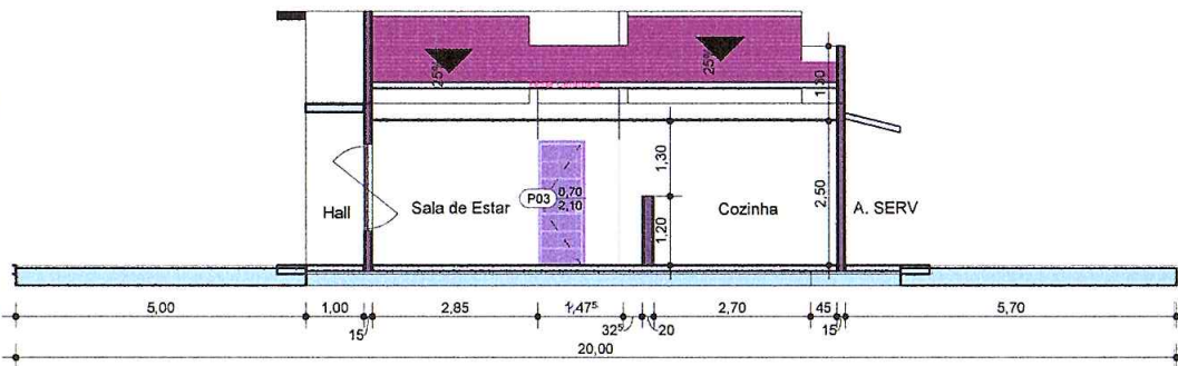
1 CORTE BB 1 : 100
