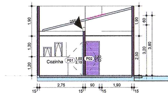
2 CORTE AA 1 : 100
