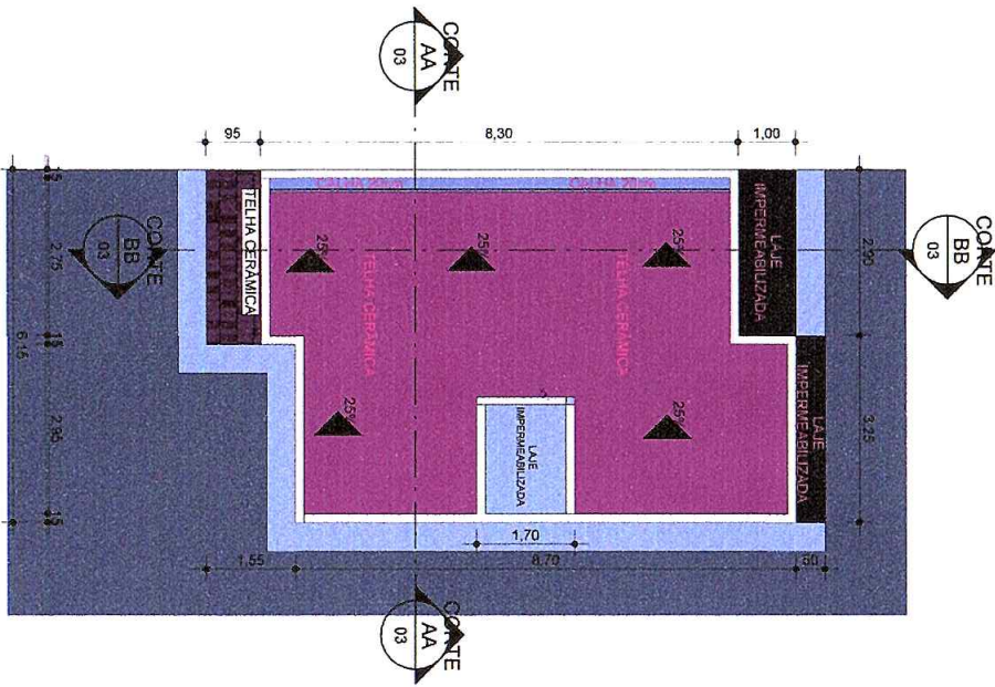
1 1 : 100 Planta de Cobertura
