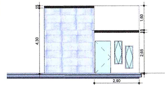
3 FACHADA FRONTAL 1 : 100
